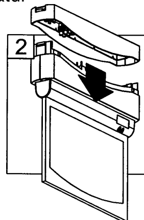
2. Dra armaturen nedåt samtidigt som clipsen hålls intryckta. Tänk på att inkopplingsplinten är spänningssatt om nätet ej bortkopplats.
