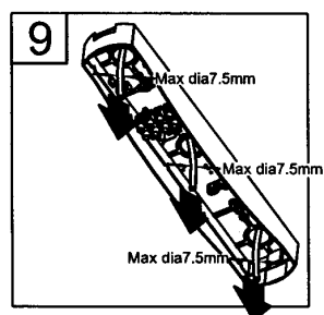
9. Dra in kabeln i takfästet.
