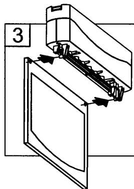
3. Montera frontskivan med framsidan mot armaturens Indikeringsdioder.
