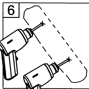
6. Borra hål i taket för fästsruvarna.
