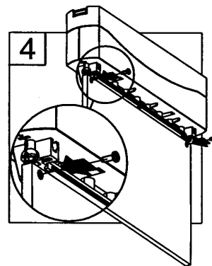
4. Lås fronten med de 2 st bifogade skruvarna.
