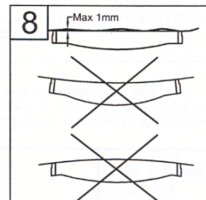
8. Taket måste vara plant för att armaturen ska få kontakt med inkopplingsplinten.
