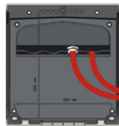
Kabelinföring baksida
